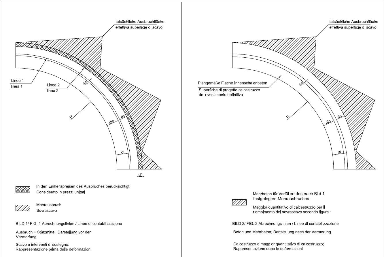
Abbildung 1 Abrechnungslinien, vor der Verformung
